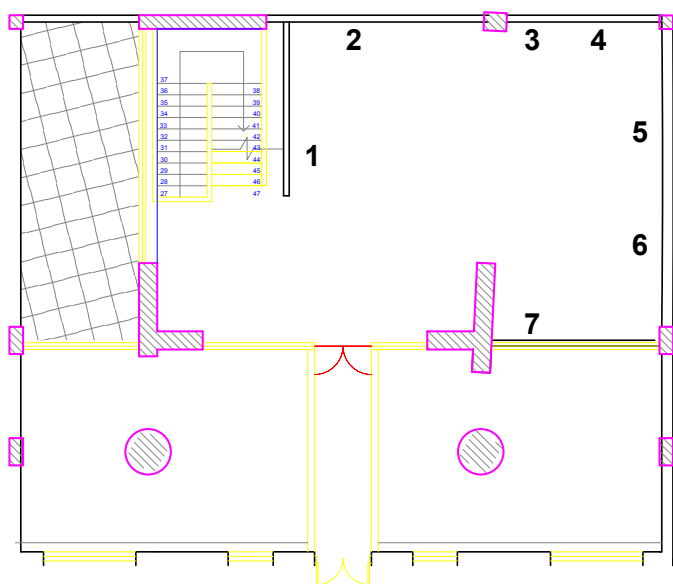
Segundo piso
